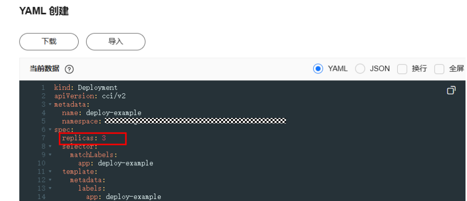
图 3-1 通过 YAML 设置工作负载实例数量
